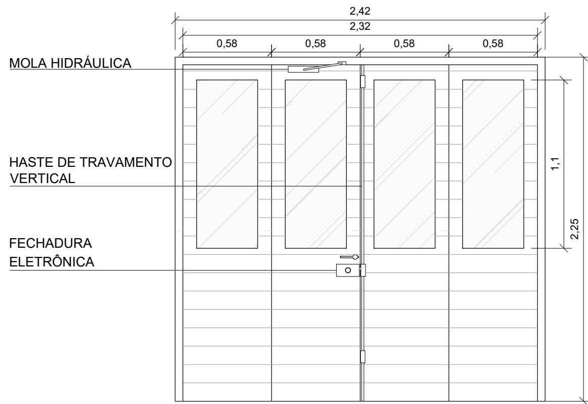
2 - ELEVAÇÃO FRONTAL
