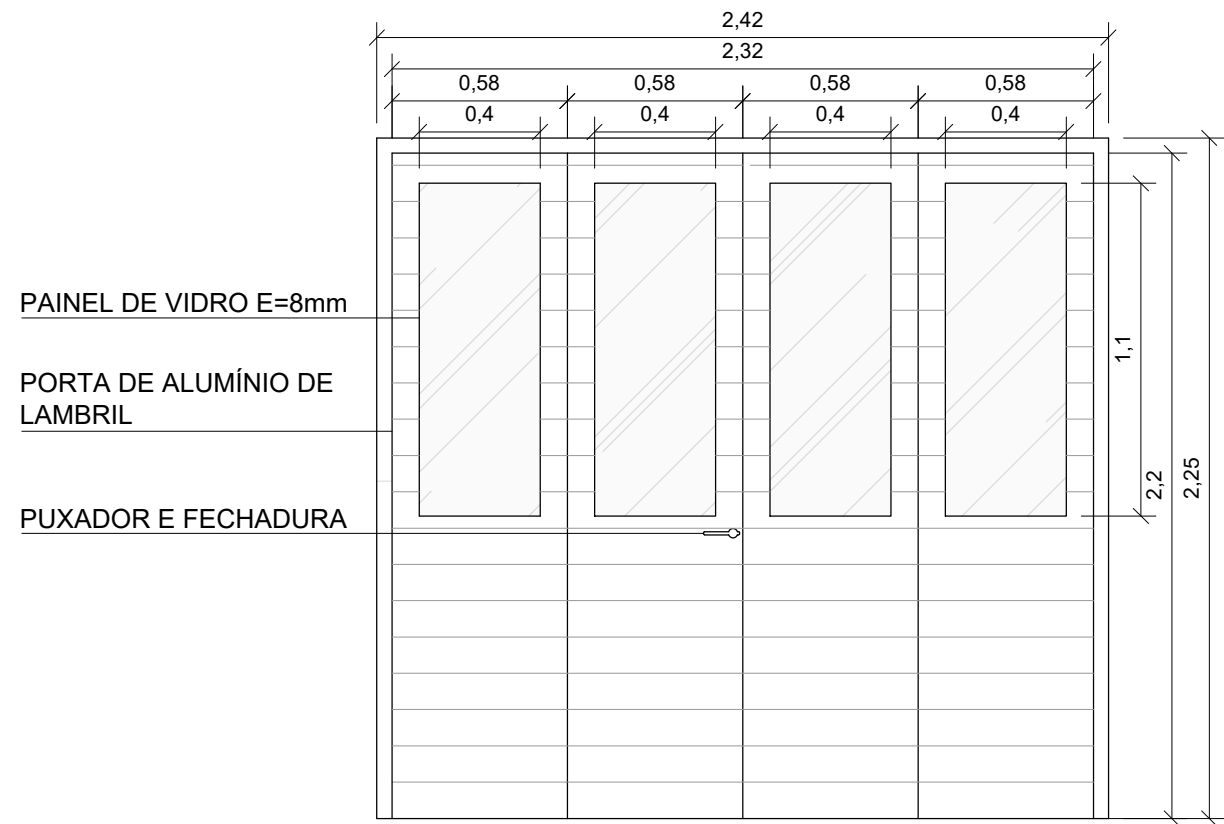
3 - ELEVAÇÃO POSTERIOR
