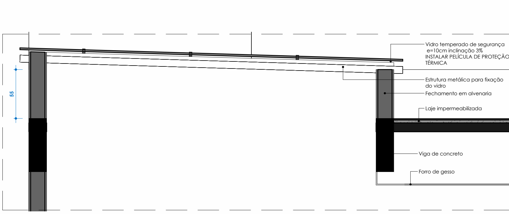
DETALHE CLARABOIA ESCADA ESC: 1 : 25
