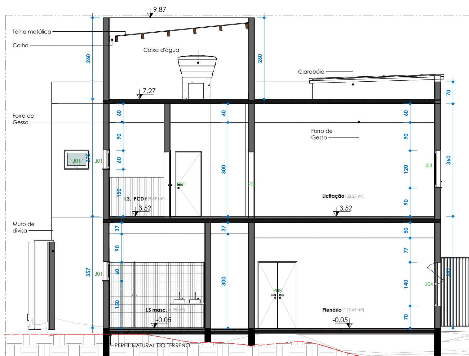
CORTE FF ESC:1 : 75
