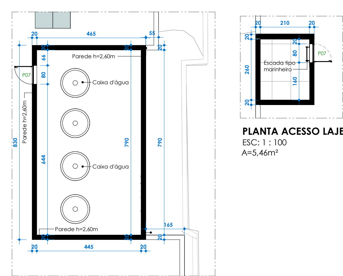
PLANTA ACESSO LAJE ESC: 1 : 100 A=5,46m²
