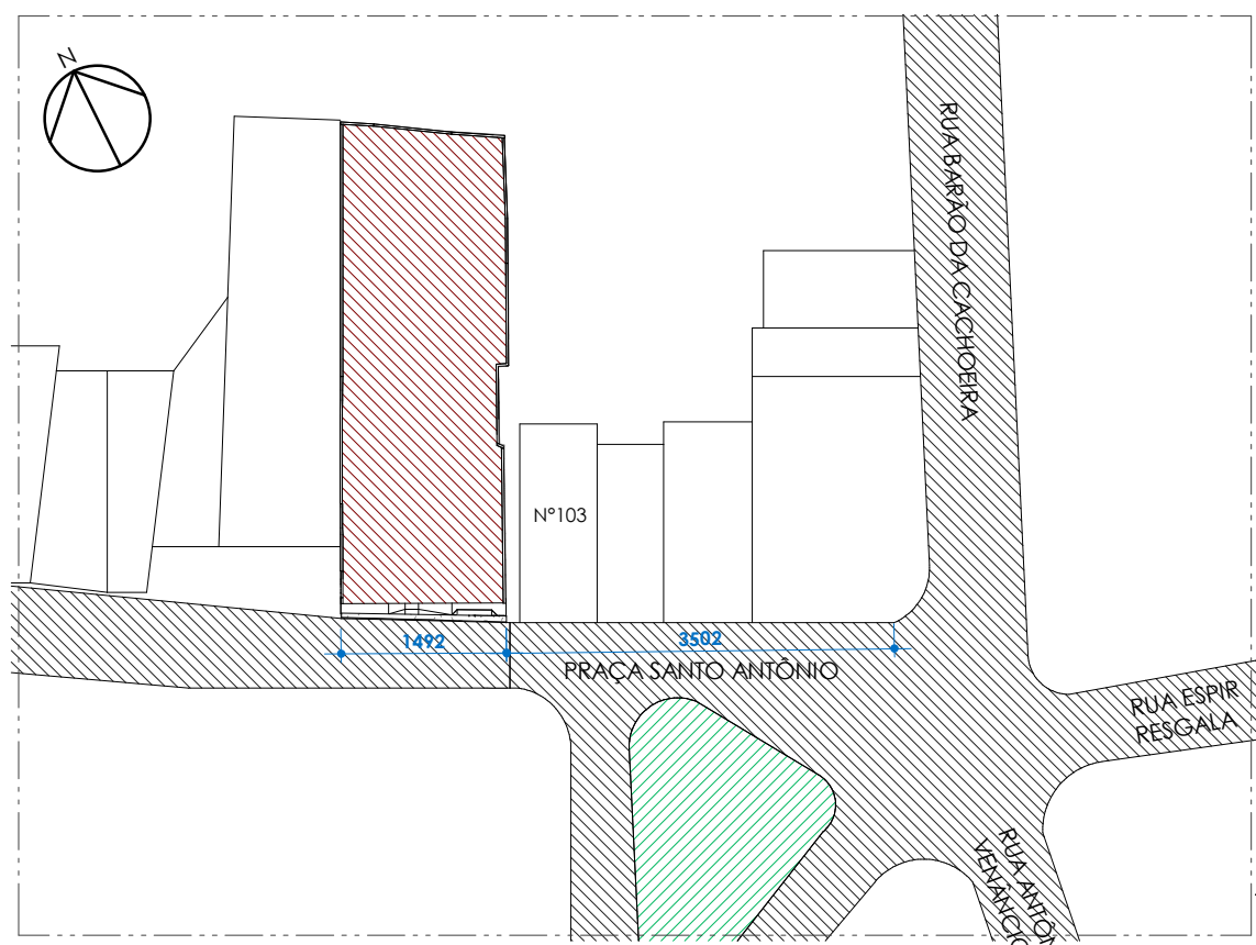
SITUAÇÃO ESC: 1 : 750
