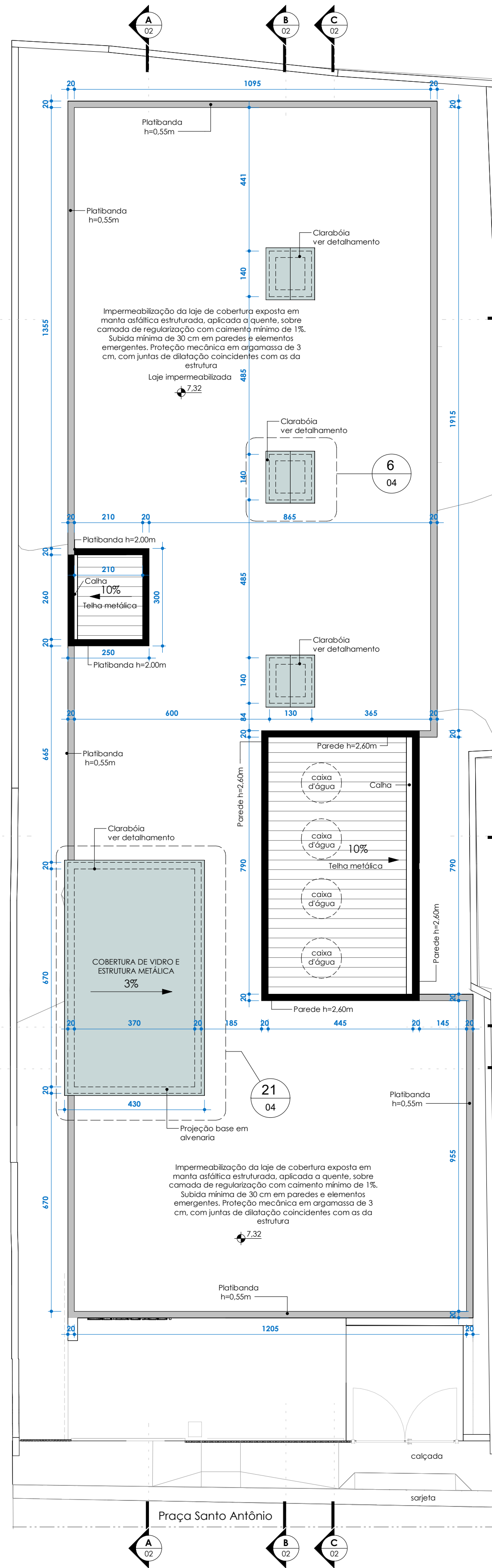
PLANTA DE COBERTURA ESC: 1 : 100
