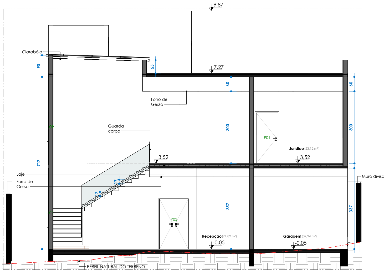
CORTE DD ESC:1 : 75
