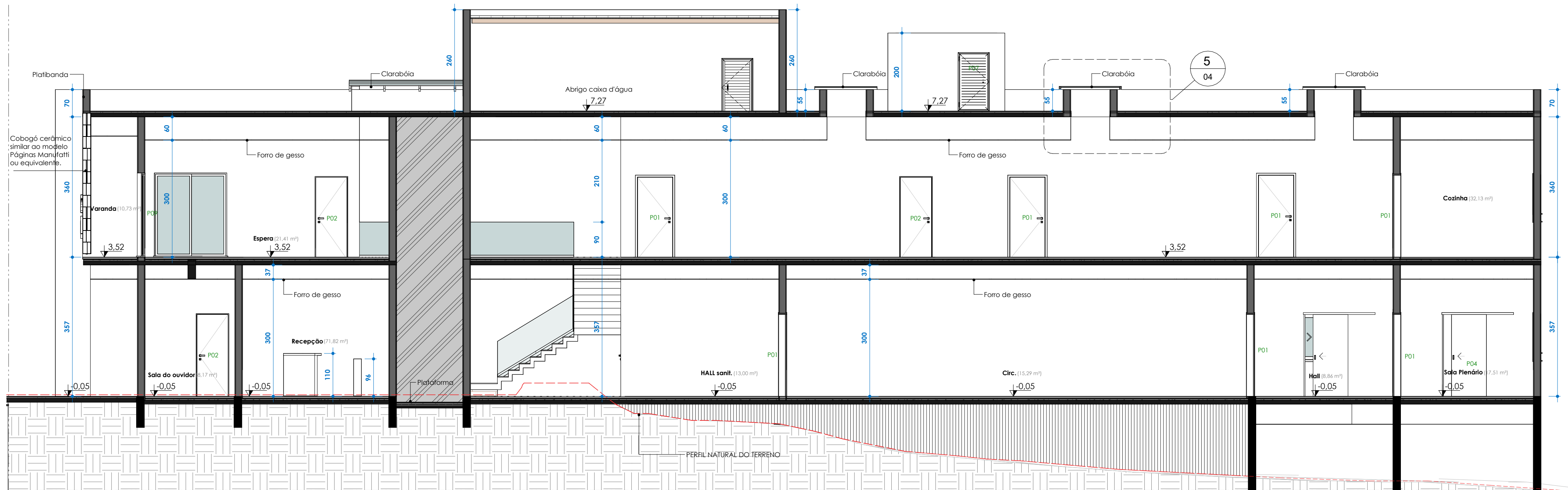
CORTE BB ESC:1 : 75
