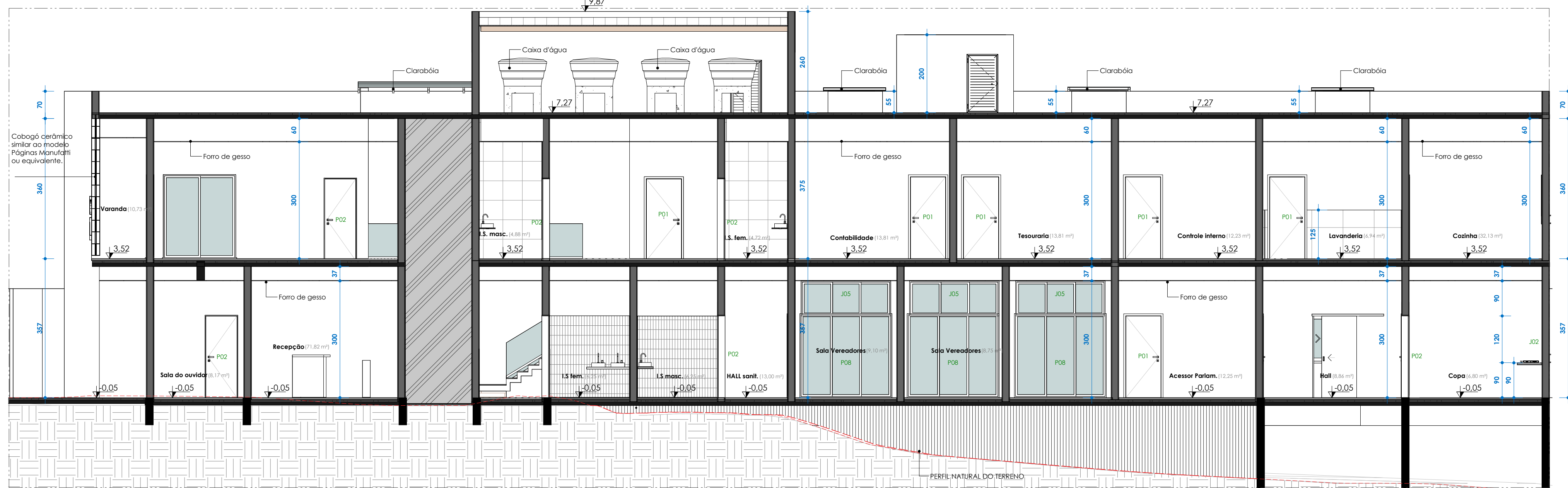
CORTE CC ESC:1 : 75
