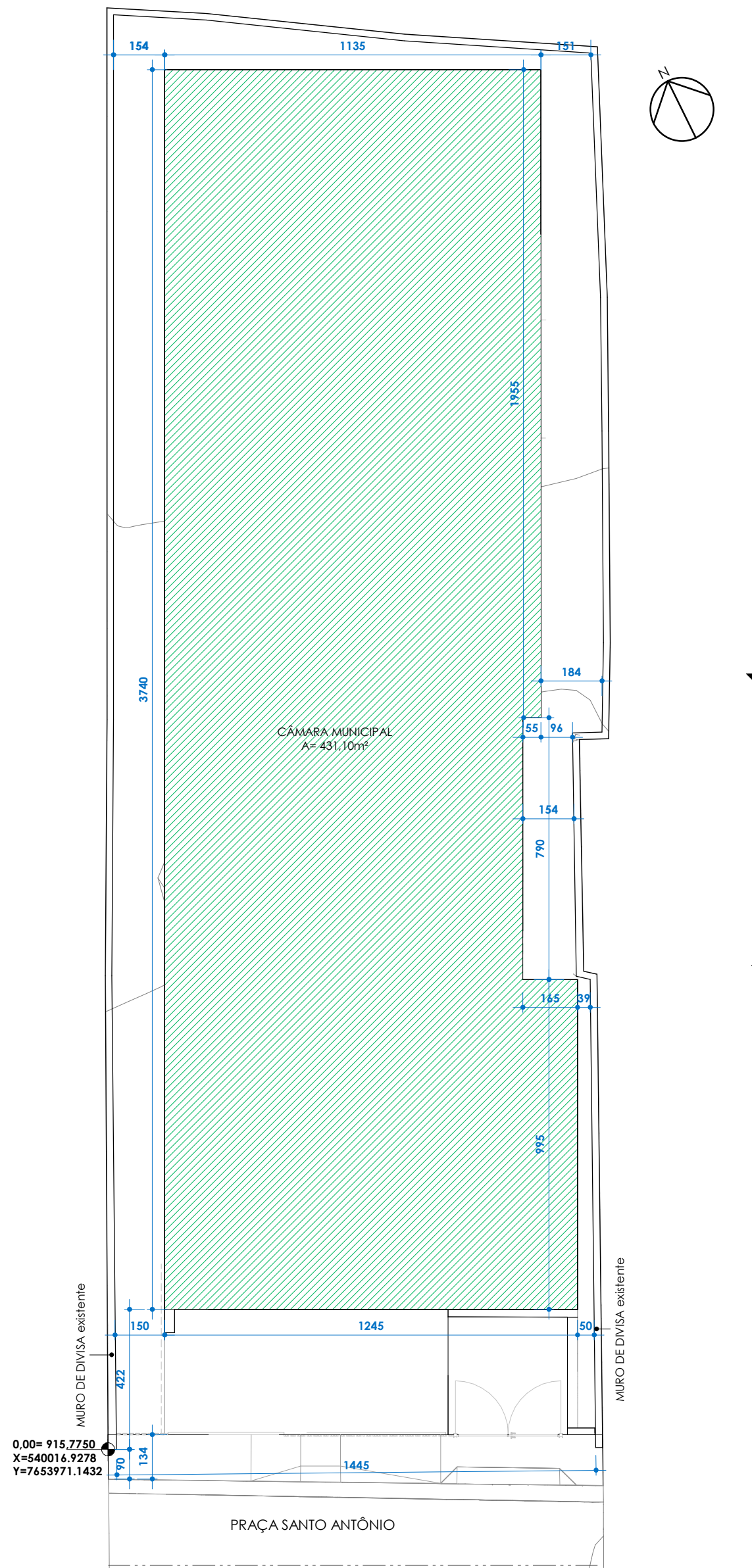
IMPLANTAÇÃO ESC: 1 : 150
