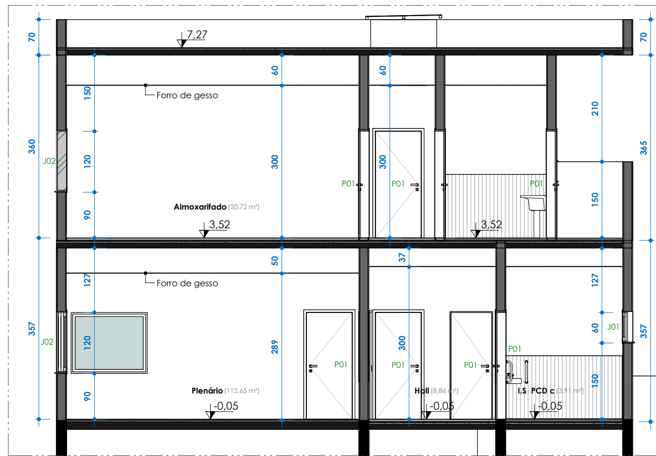
CORTE GG ESC:1 : 75
