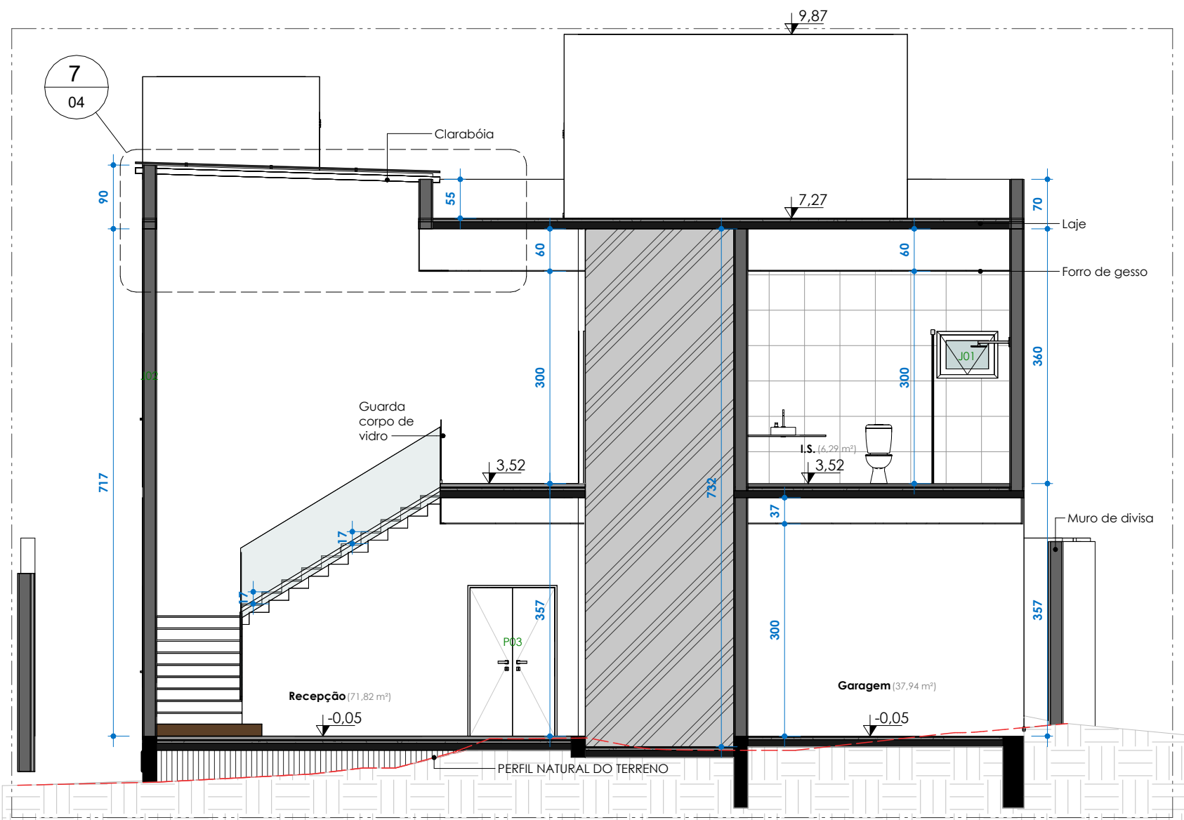
CORTE EE ESC:1 : 75
