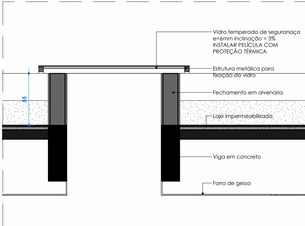
DETALHE CLARABOIA CORREDOR ESC: 1 : 25
