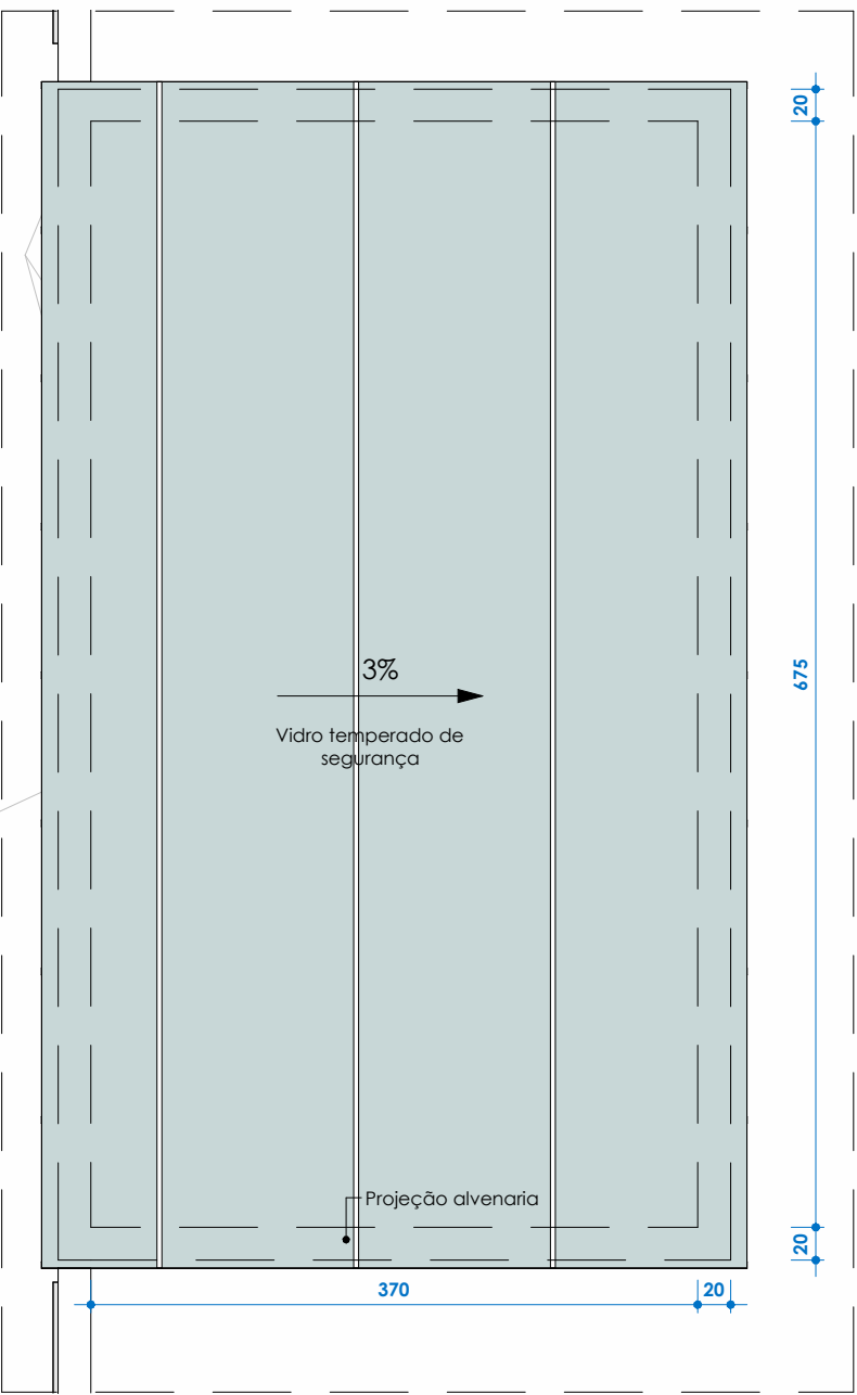
PLANTA CLARABOIA ESCADA ESC: 1 : 50
