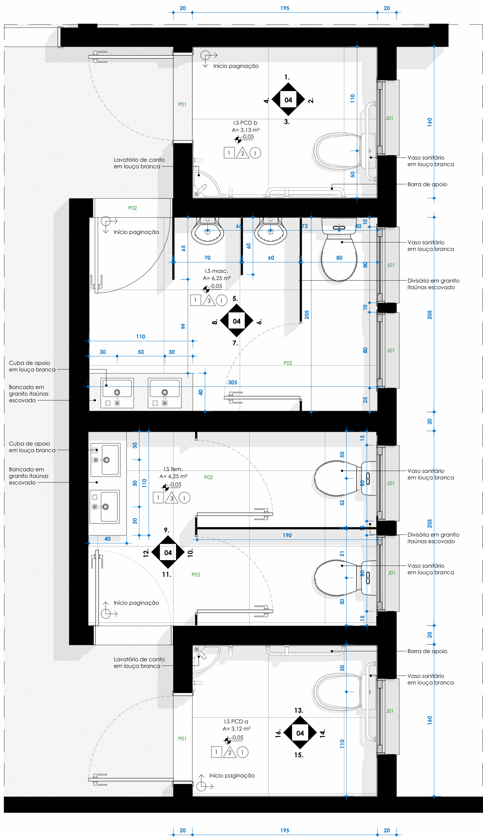
PLANTA BAIXA BANHEIROS PÁV. TÉRREO- USO PÚBLICO ESC: 1 : 25
