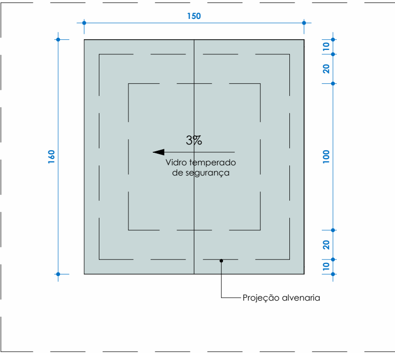
PLANTA CLARABOIA CORREDOR ESC: 1 : 25
