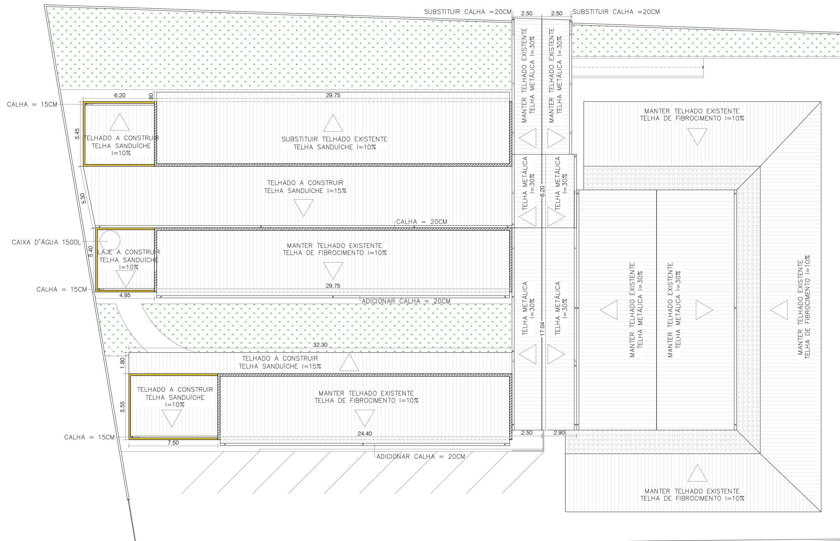
PLANTA DE COBERTURA ESCALA MEDIDAS EM METROS
