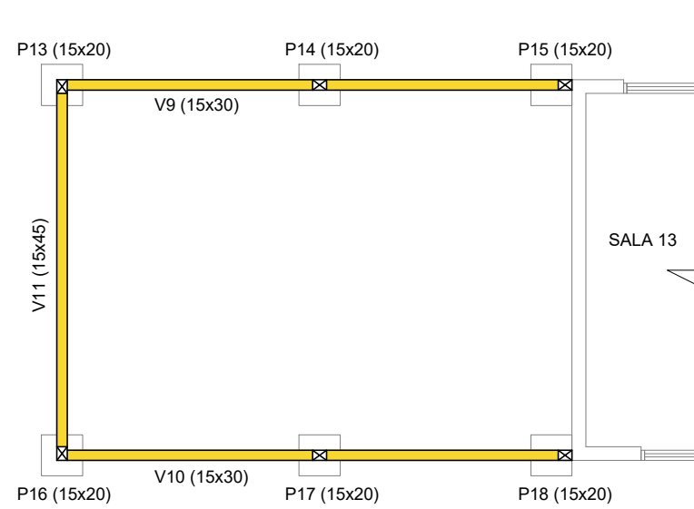
LOCAÇÃO ESTRUTURAL ESCALA MEDIDAS EM METROS
