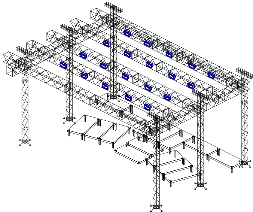
VISTA PERSPECTIVA
