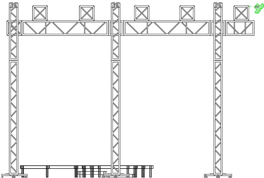
VISTA LATERAL
