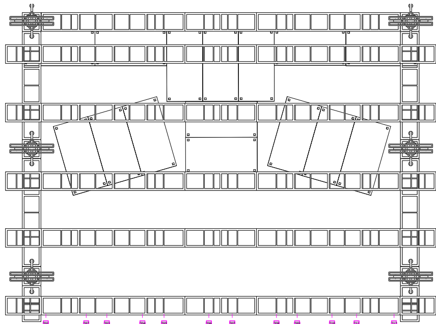
VISTA TETO
