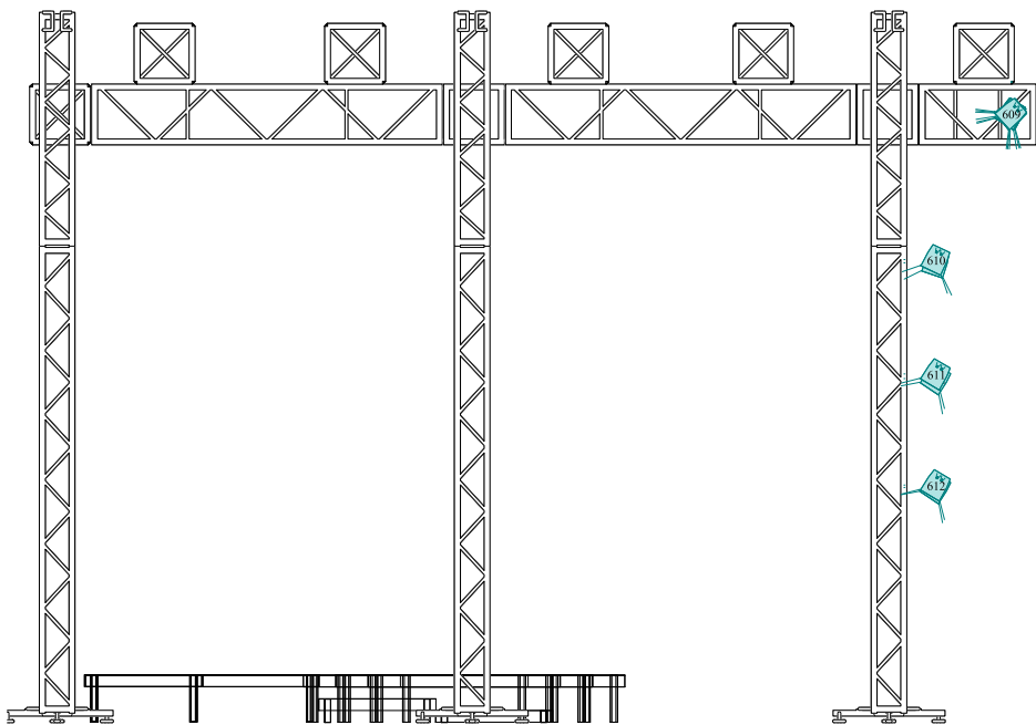
VISTA LATERAL
