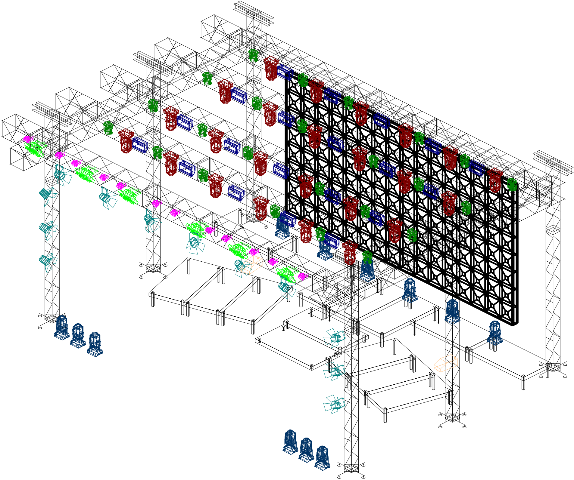
VISTA PERSPECTIVA
