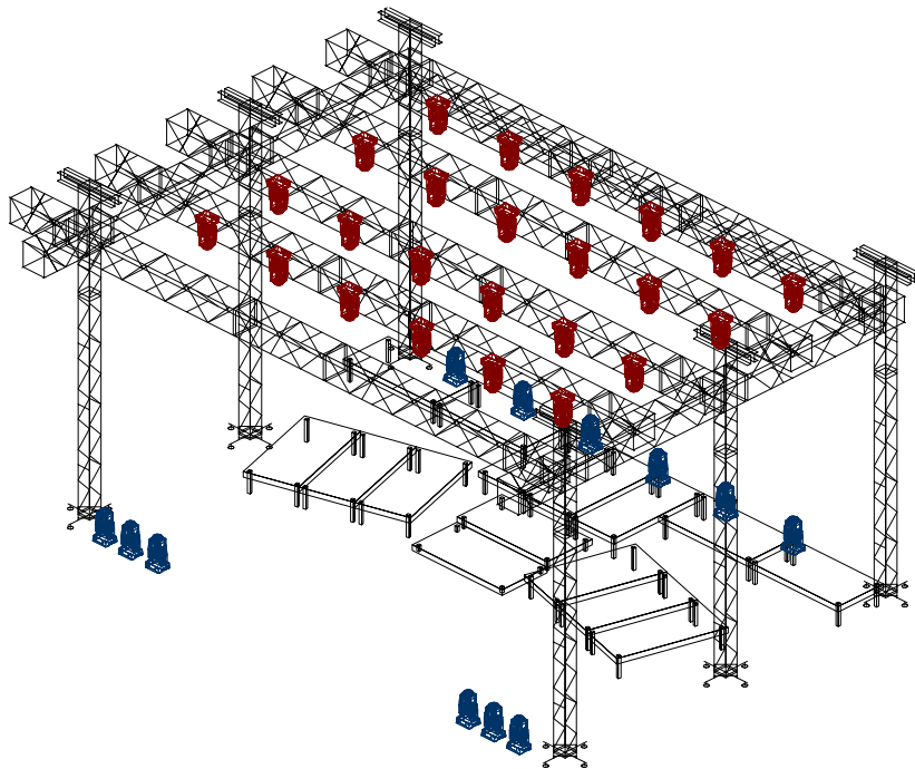
VISTA PERSPECTIVA
