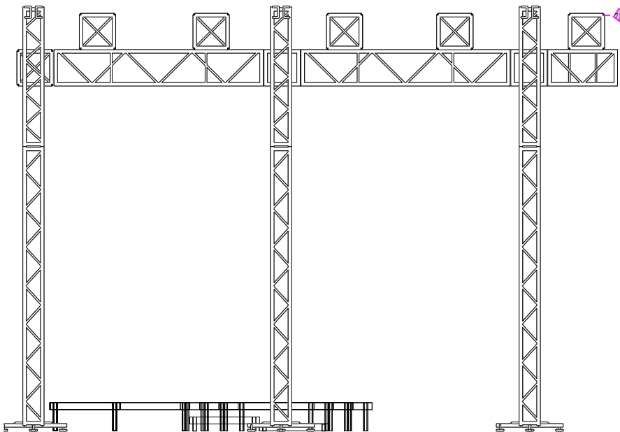
VISTA LATERAL
