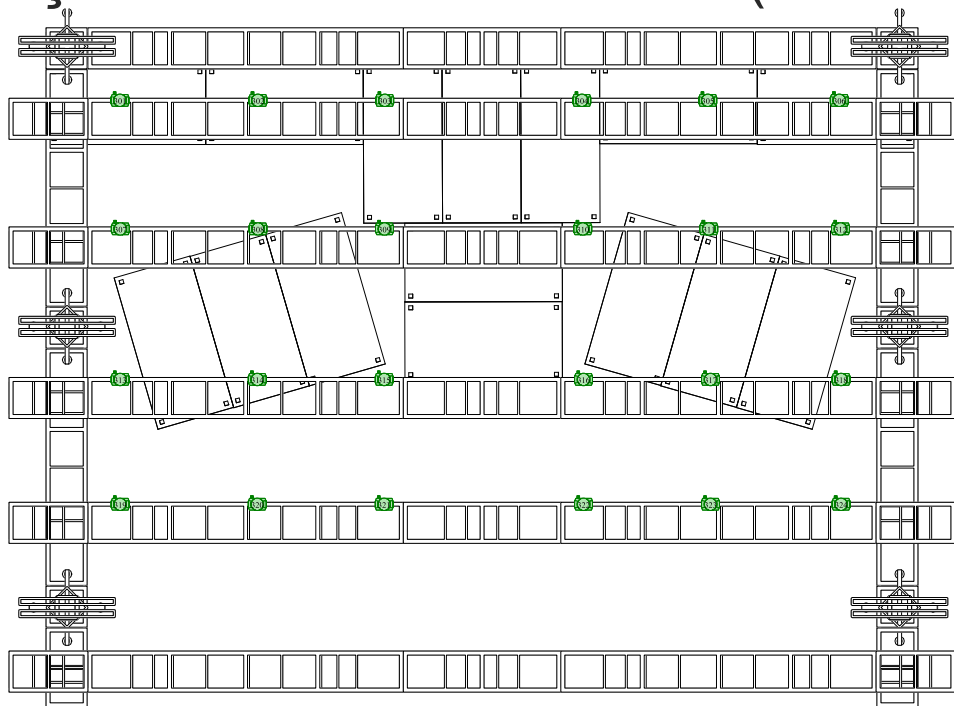
VISTA TETO
