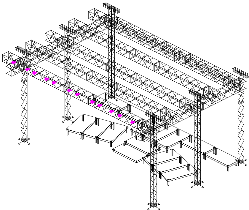
VISTA PERSPECTIVA
