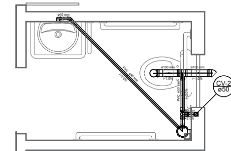
Detalhe S2 escala 1:25
