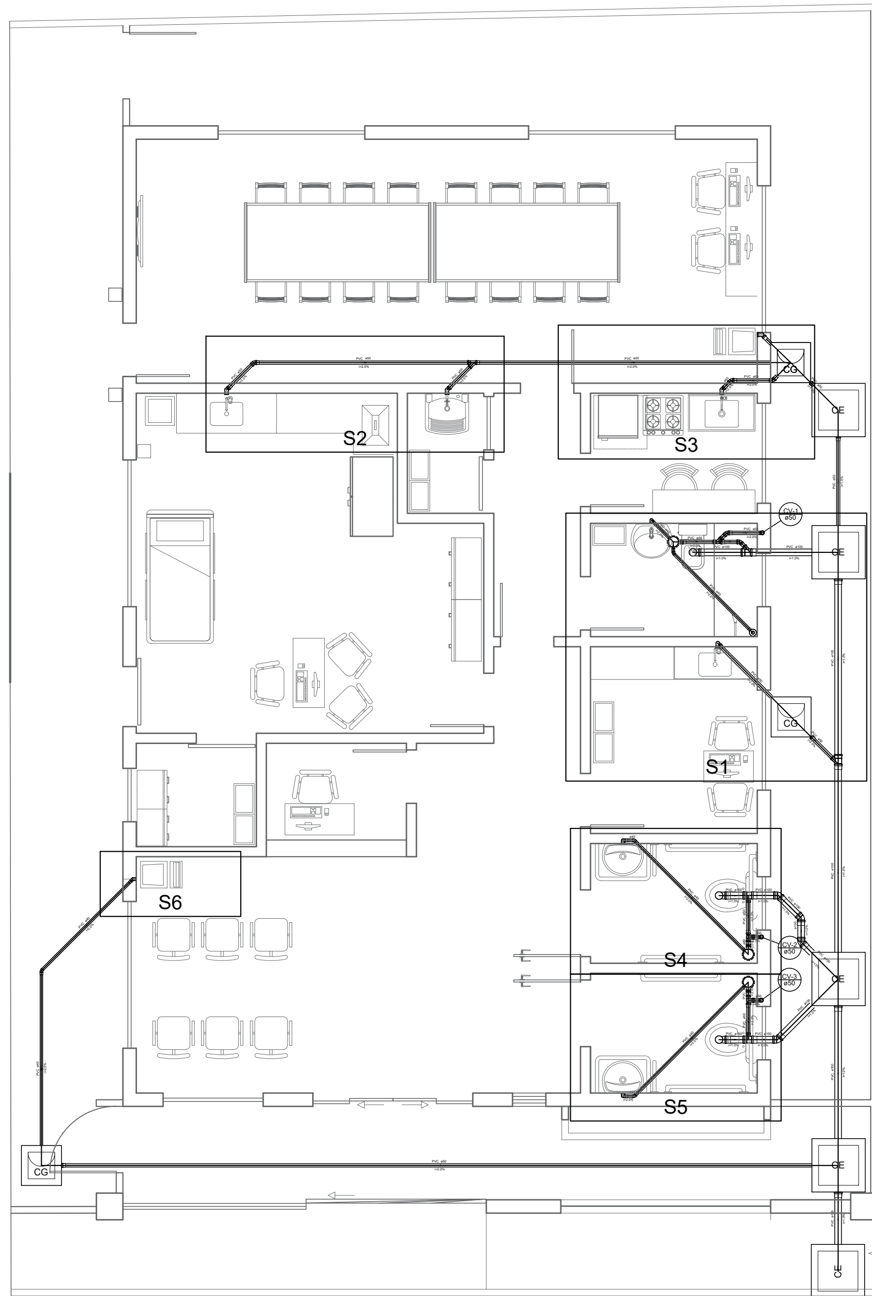
PLANTA BAIXA ESGOTO TERREO Escala 1:75
