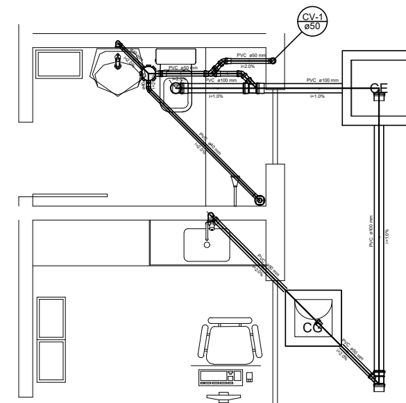
Detalhe S1 escala 1:25
