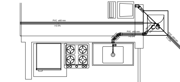
Detalhe S6 escala 1:25
