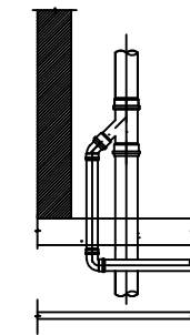
Detalhe S3 escala 1:25
