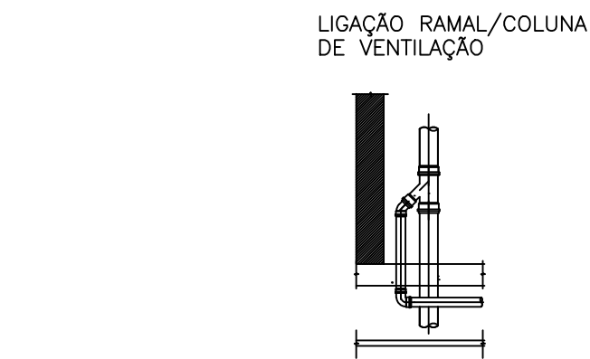
Detalhe S3 escala 1:25
