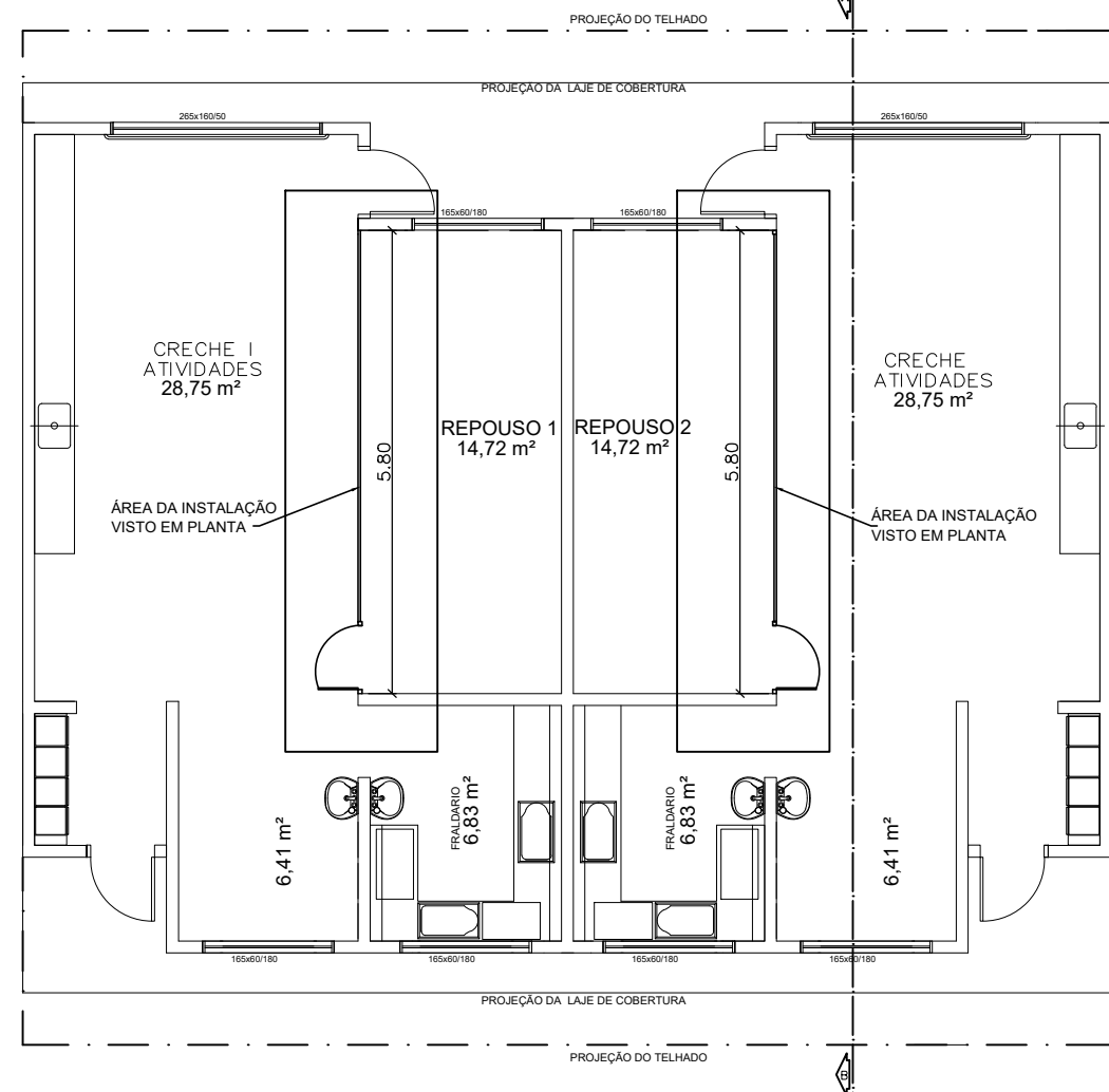
1 PLANTA BAIXA ÁREA TOTAL = 131,61 M 2
