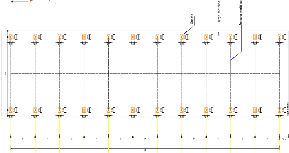
PLANTA BAIXA
