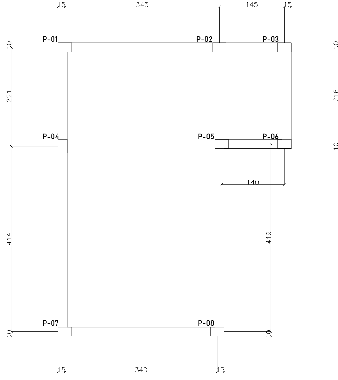
Locação de Pilares
