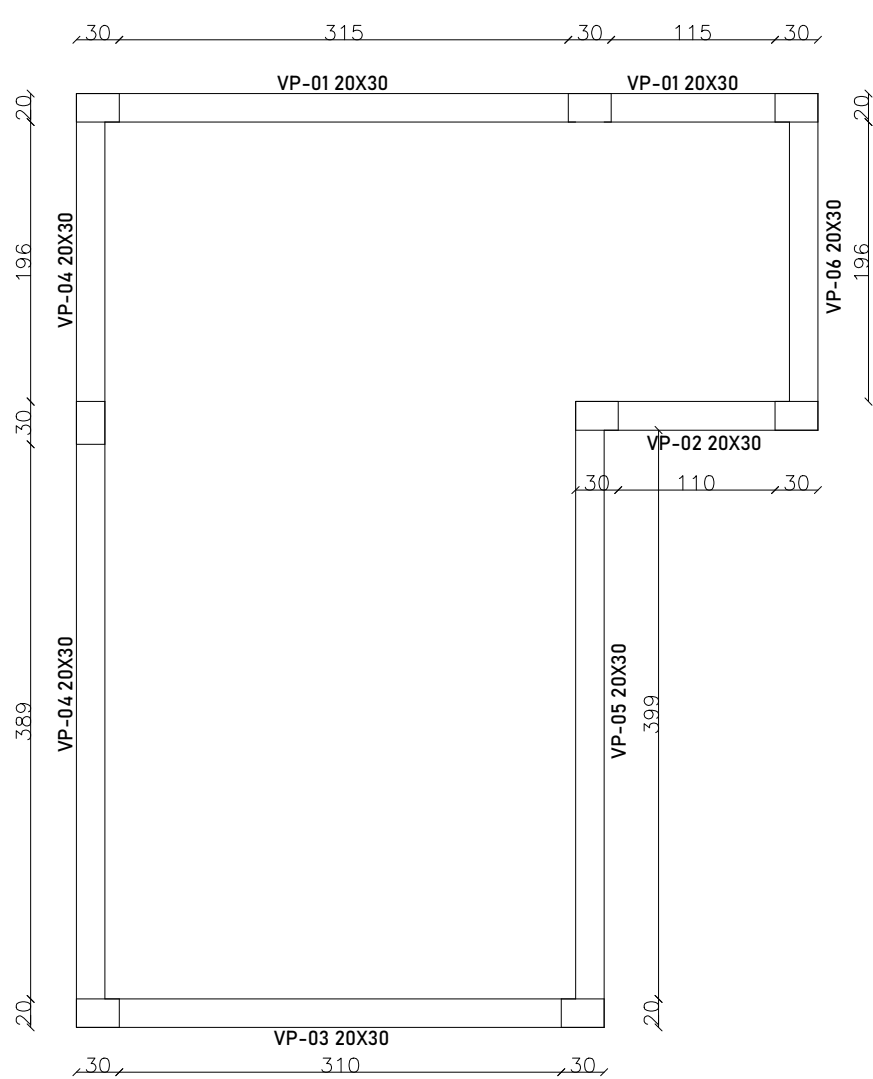
Locação Viga Platibanda
