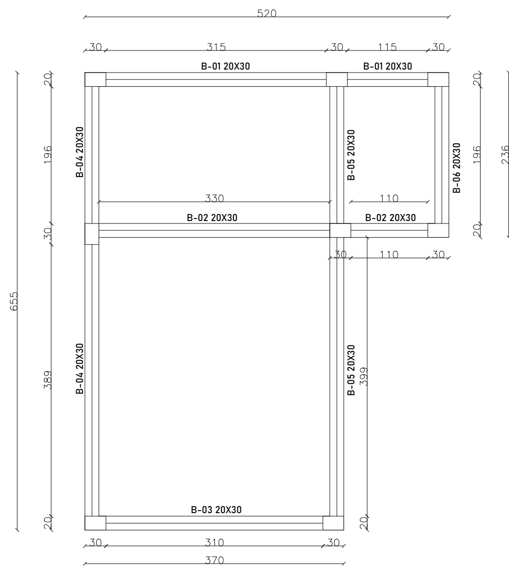
Locação de Baldrames
