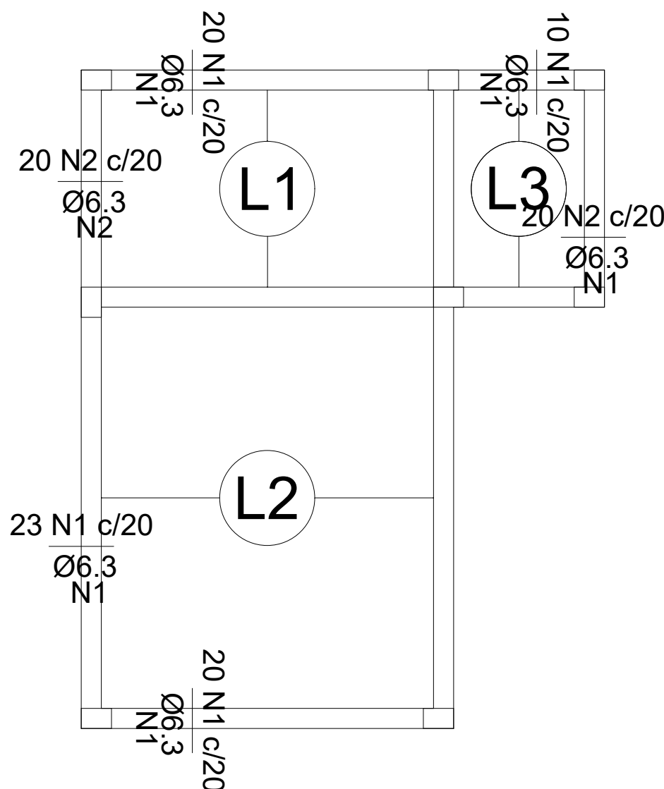
Armação Negativa Laje
