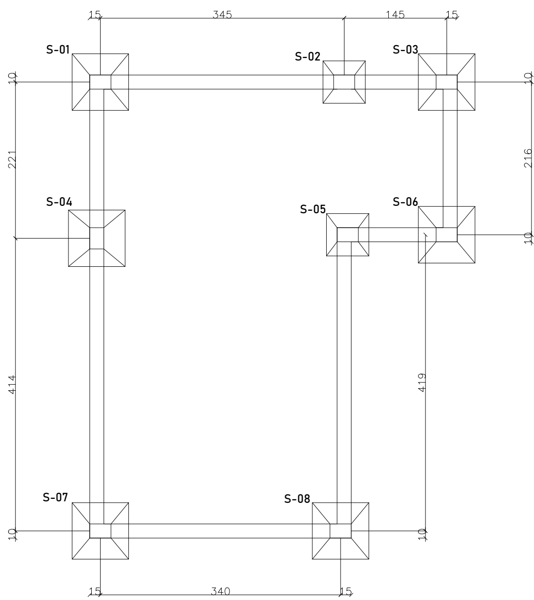
Locação de Sapatas
