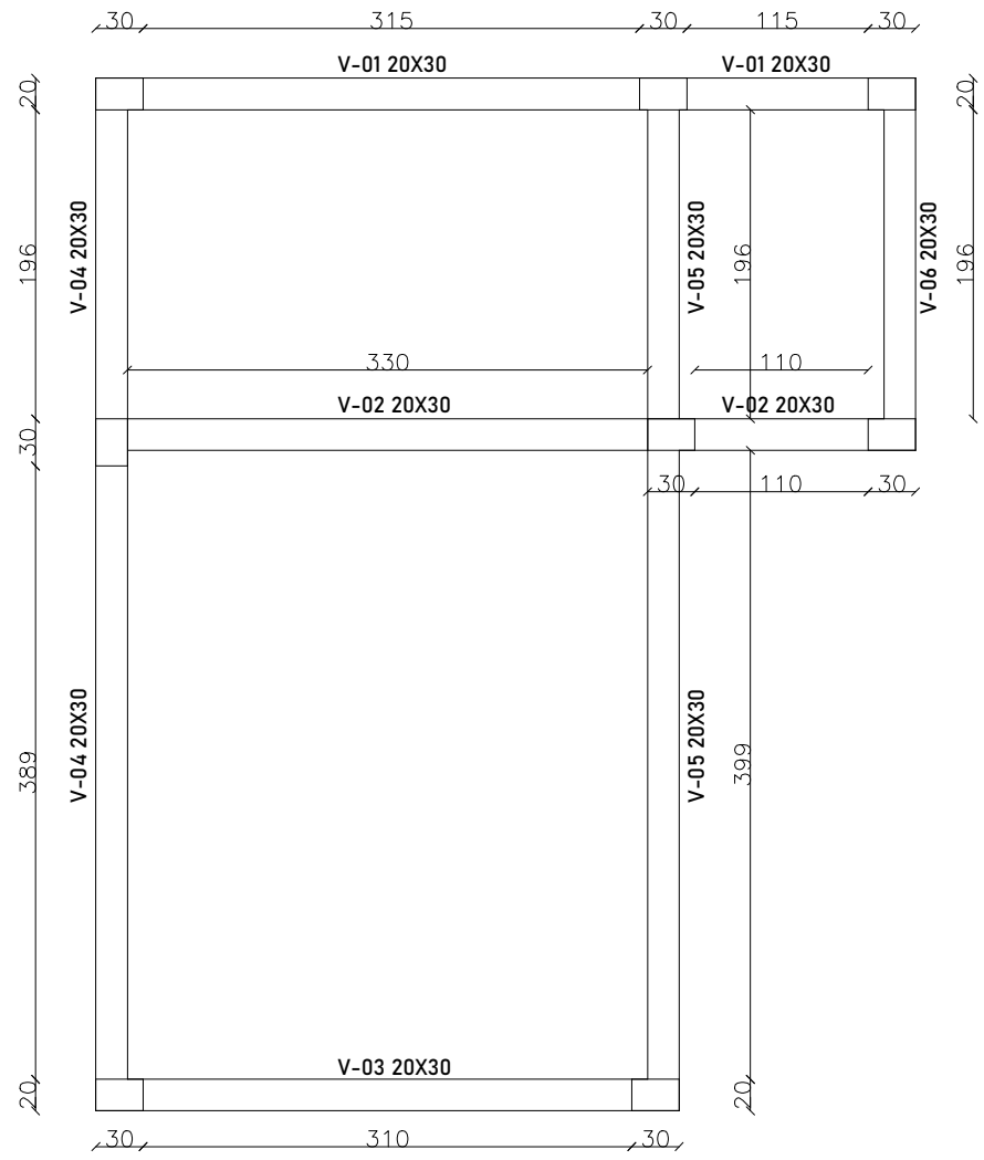
Locação de Vigas
