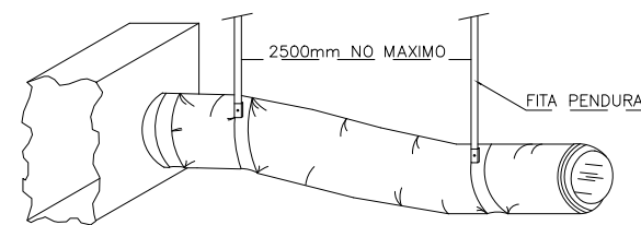
FIXAÇÃO E SUPORTE DO DUTO FLEXÍVEL. 5/ESCALA
