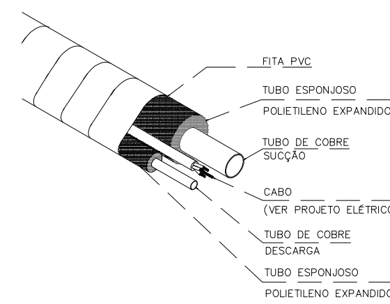
LINHAS FRIGORÍGENAS E DRENO. 5/ESCALA
