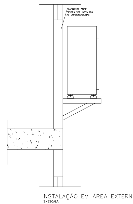
INSTALAÇÃO EM ÁREA EXTERNA. 5/ESCALA
