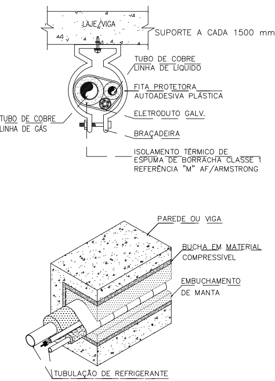
FIXAÇÃO DAS LINHAS FRIGORÍGENAS. 5/ESCALA
