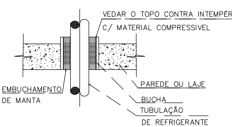
BUCHAS P/ PASSAGEM DAS TUBULAÇÕES DE COBRE EM LAJE OU ALVENARIA. 5/ESCALA
