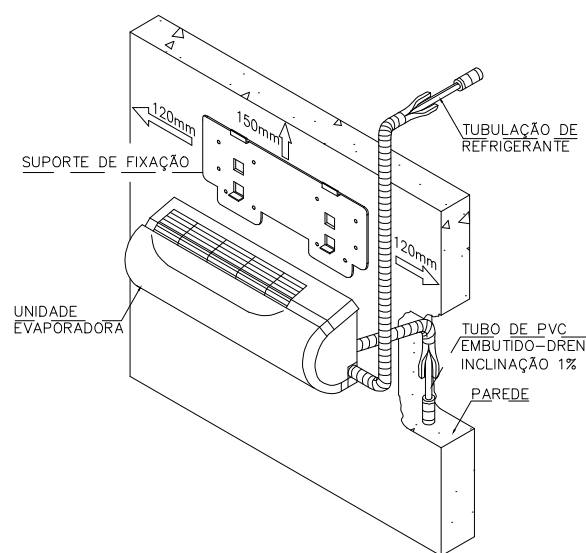
EVAPORADOR HI WALL. 5/ESCALA
