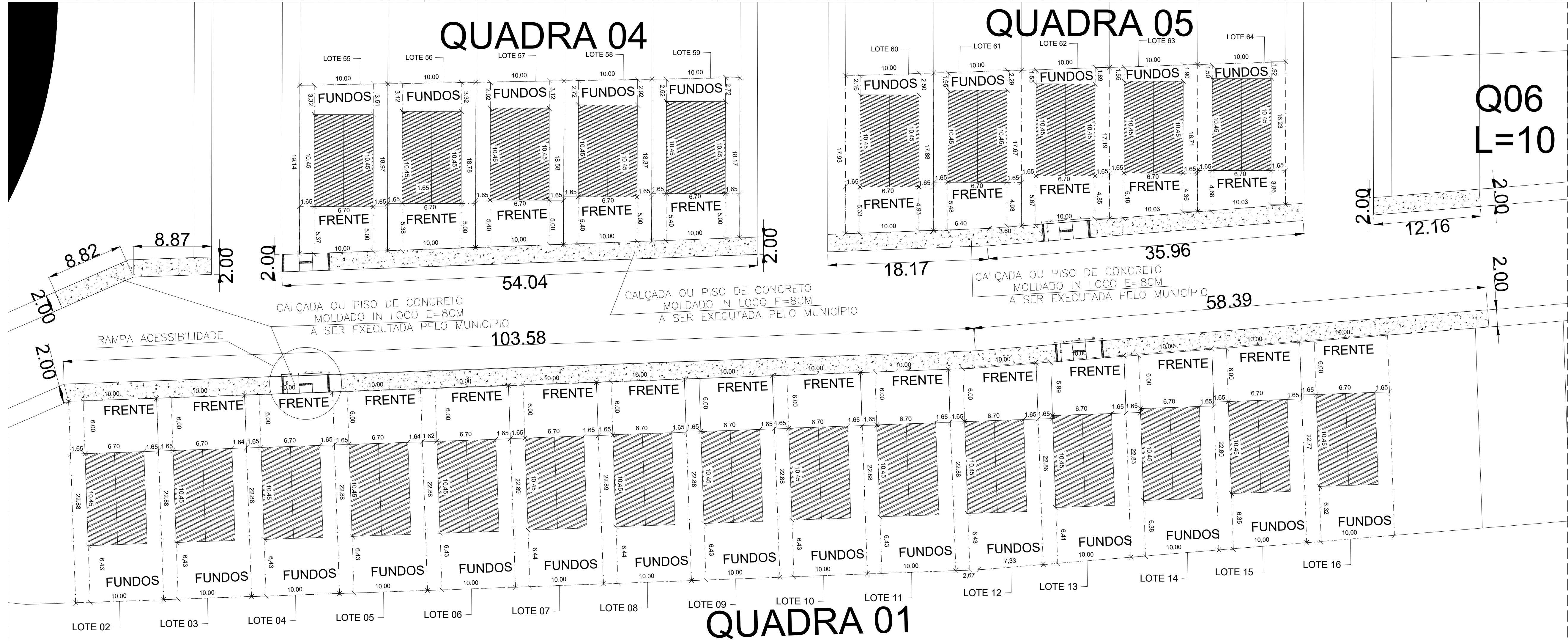
DETALHE ÁREA DE IMPLANTAÇÃO UNIDADE HABITACIONAL
