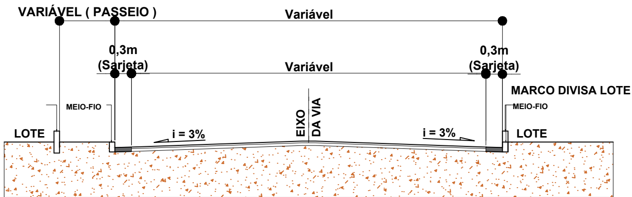
SEÇÃO TRANSVERSAL TIPO DAS RUAS
