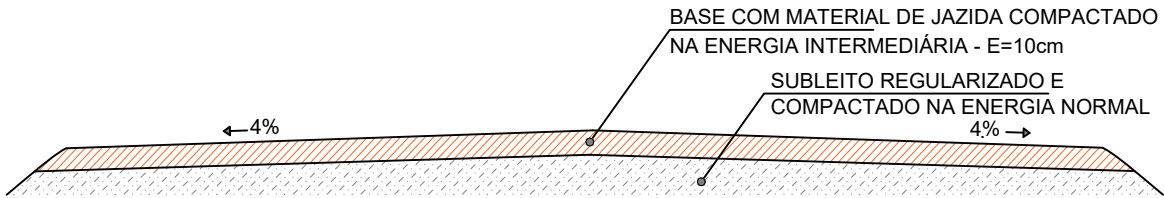
DETALHE 1 PISTA PRINCIPAL
