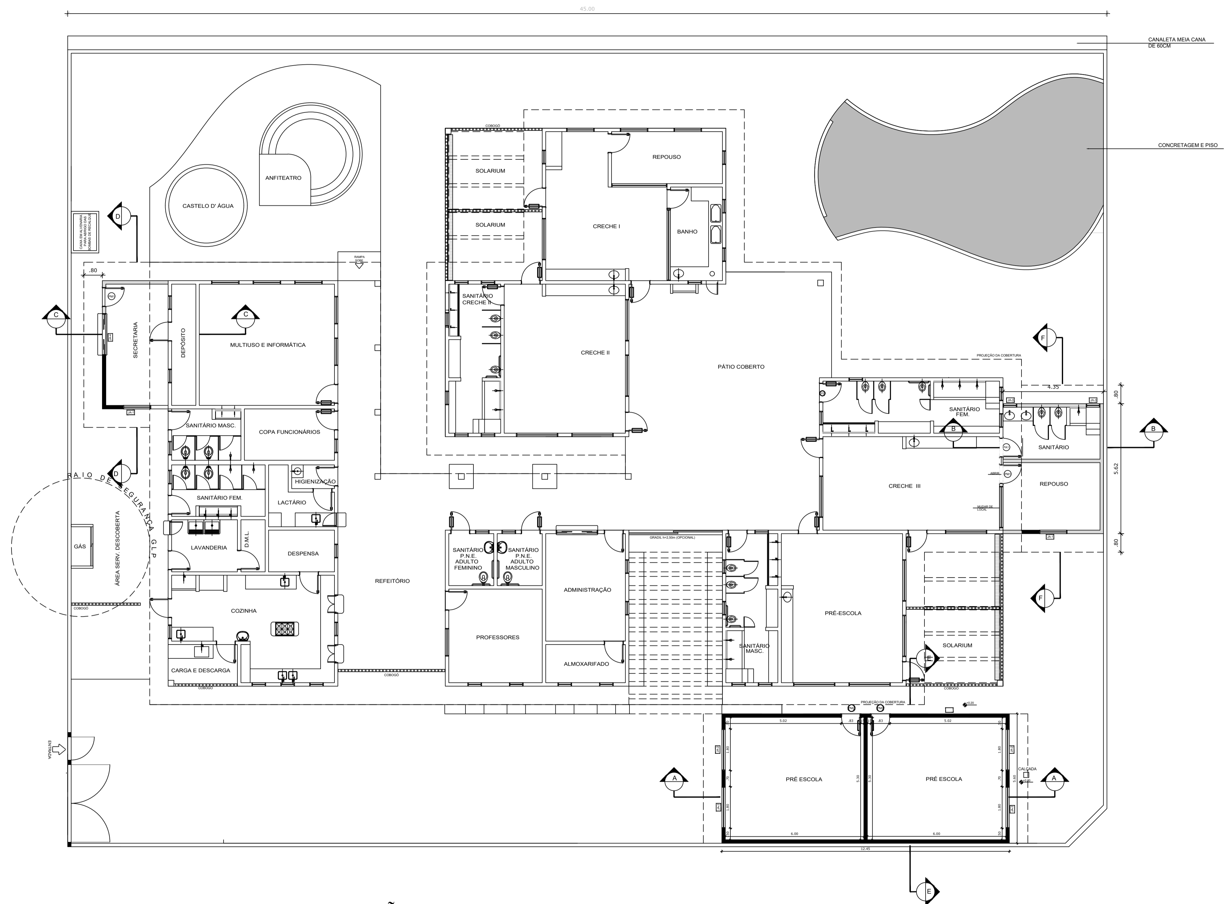
PLANTA BAIXA GERAL E LOCAÇÃO
