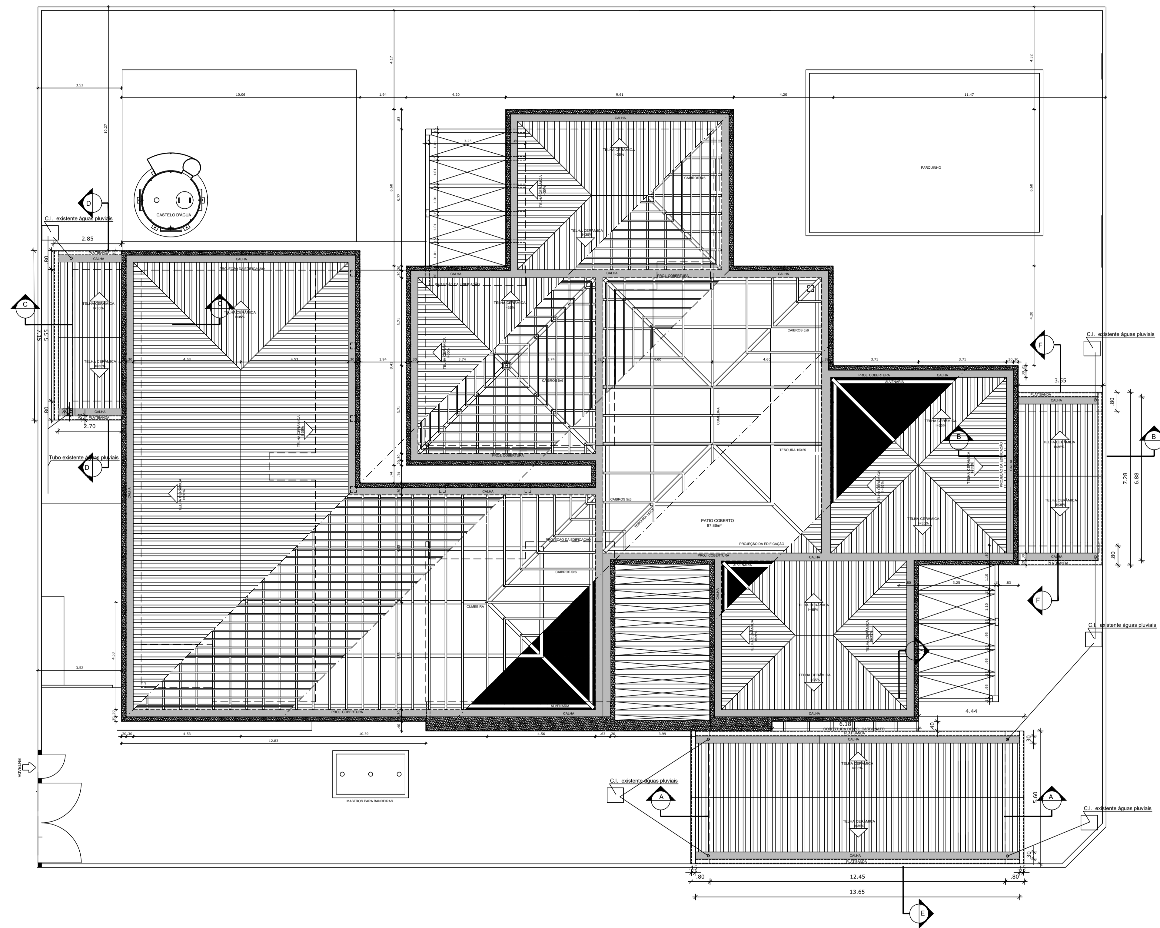
PLANTA DE COBERTURA
