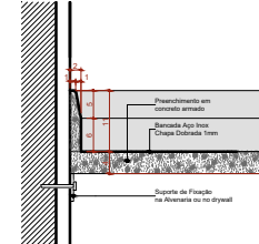
Det. B.1a Bancada de Inox Detalhe Frontão - Área Molhada Escala 1:5
