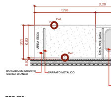
BPC.220e Escala 1:20
