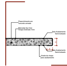
Det. B.1d Bancada de Inox Detalhe Sala - Área Seca Escala 1:5
