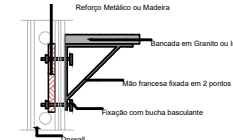
DET REFORÇO DRYWALL Escala 1:20
