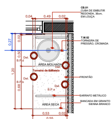
BPC.120e Escala 1:20
