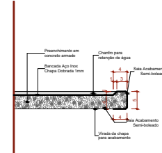
Det. B.1b Bancada de Inox Detalhe Sala - Área Molhada Escala 1:5
