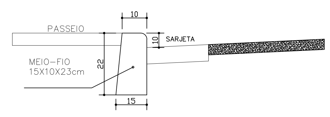
DET. (MEIO-FIO E PASSEIO) SEM ESCALA - MEDIDAS EM CENTIMETROS
